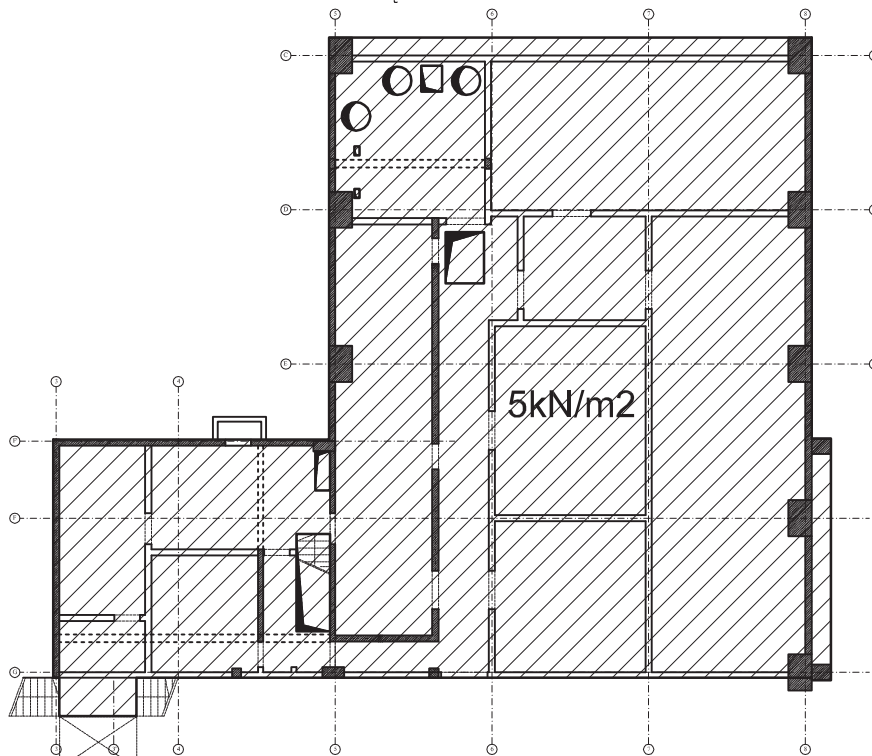
STROP NAD PIWNICĄ (rzędna -0,10m) obciążenie zmienne
