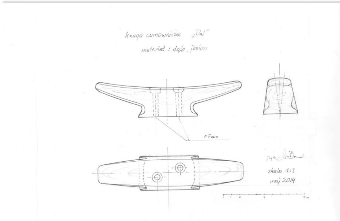
Rysunek 1: Knaga z jachtu „Dal”
