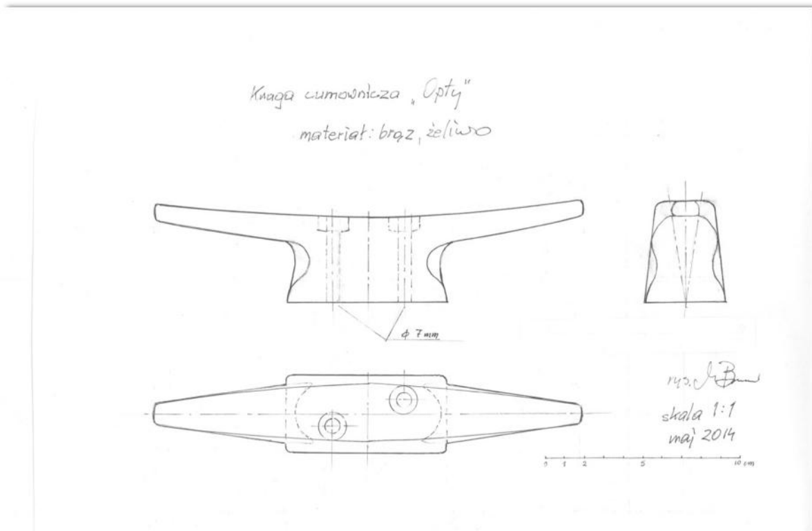
Rysunek 2: Knaga z jachtu „Opty”
